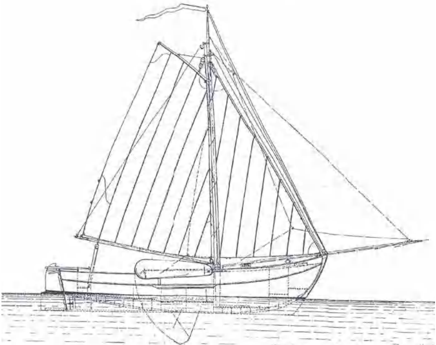
Tuigplan stalen vissloep
